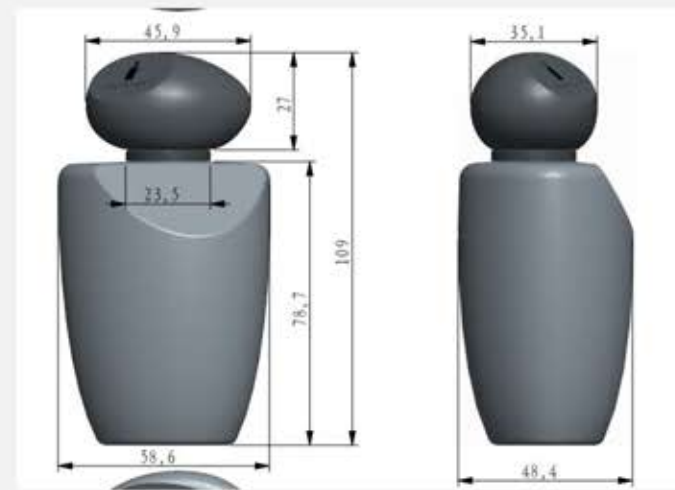
总尺寸
