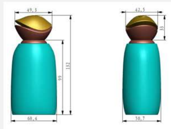
总尺寸
