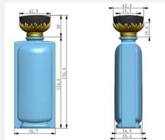
总尺寸
