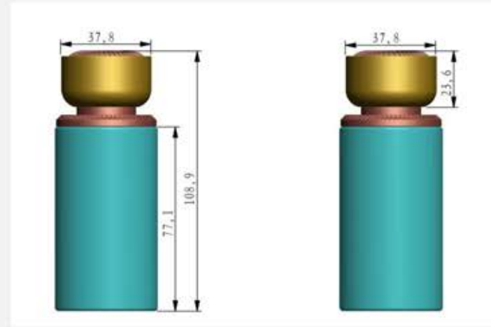
总尺寸
