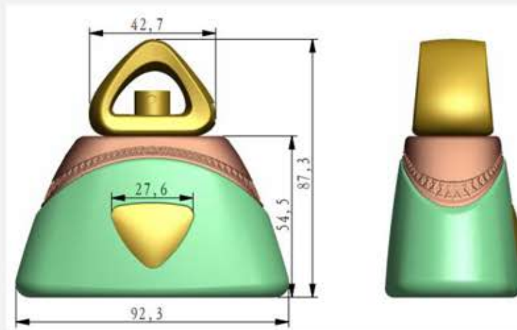
总尺寸
