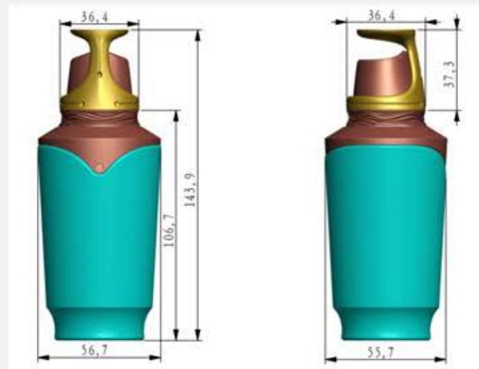
总尺寸
