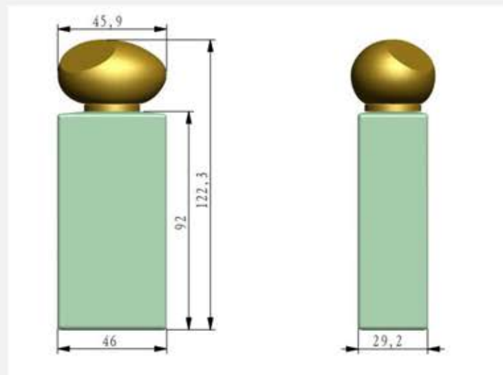
总尺寸
