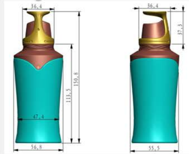
总尺寸
