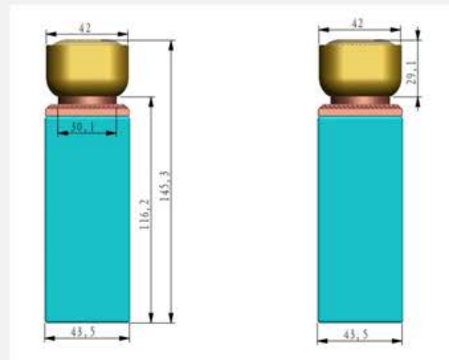
总尺寸
