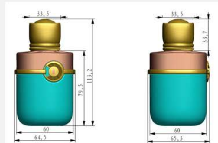
总尺寸
