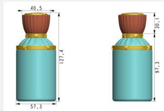
总尺寸
