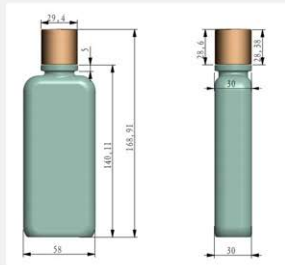
总尺寸
