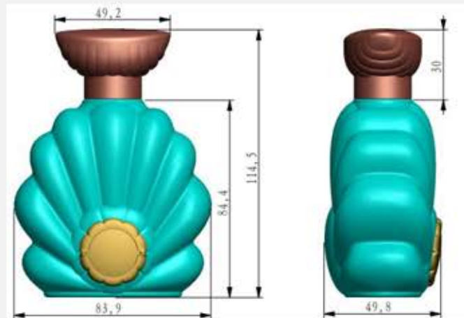
总尺寸
