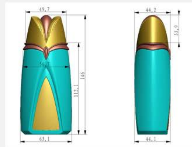
总尺寸
