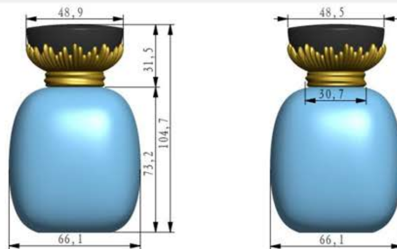
总尺寸
