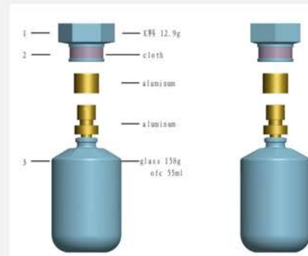
爆炸图
